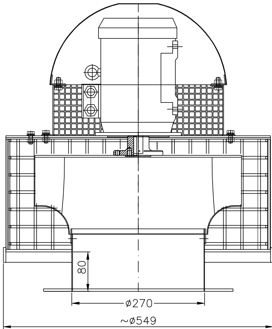
Kołnierz wlotu
